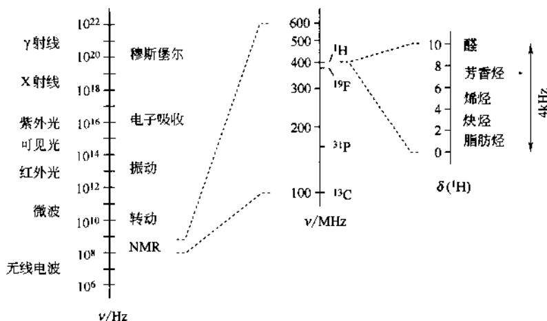
图 1.8 电磁谱及磁场 ( B=9.4 T) 中一些原子核的核磁共振频率和 ^1\text{H} 的化学位移
