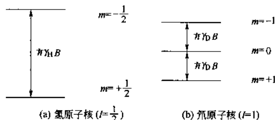
图 1.7 氢原子核 ( I = \frac{1}{2} ) 和氘原子核 ( I = 1 ) 在磁场 (大小为 B ) 中的能级
