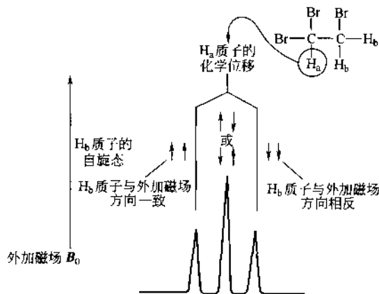
图 1.12 ^1\text{H} NMR 中质子的耦合示例
