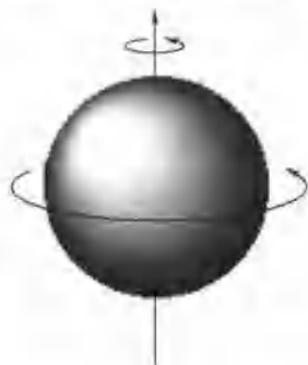
图 1.1 质子自旋电荷产生的磁偶极
