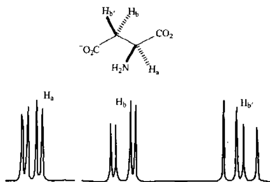
图 1.13 同碳上的两个磁不等价质子对相邻手性碳原子上质子的耦合
