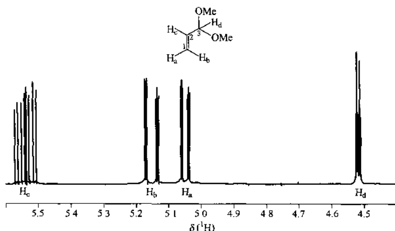
图 1.11 某烯烃衍生物的局部 ^1\text{H} NMR 谱
