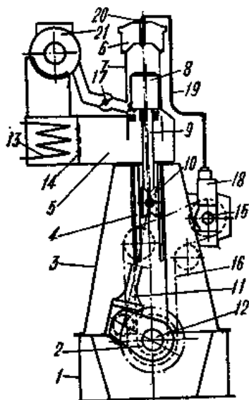
图1-2 二冲程柴油机的主要部件 1-机座; 2-主轴承; 3-机架; 4-导板; 5-扫气箱; 6-气缸盖; 7-气缸体; 8-活塞; 9-活塞杆; 10-十字头; 11-连杆; 12-曲轴; 13-空气冷却器; 14-气阀; 15-凸轮轴; 16-凸轮轴传动链; 17-排气转阀; 18-喷油泵; 19-燃油管; 20-喷油器; 21-增压器
