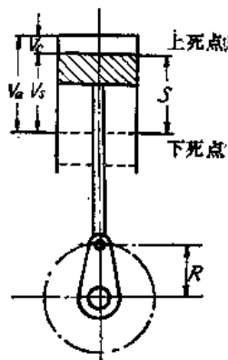
图1-3 柴油机的几何名称
