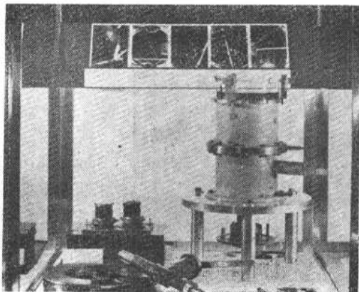
约里奥自己制造的著名的可变压威尔逊云室
