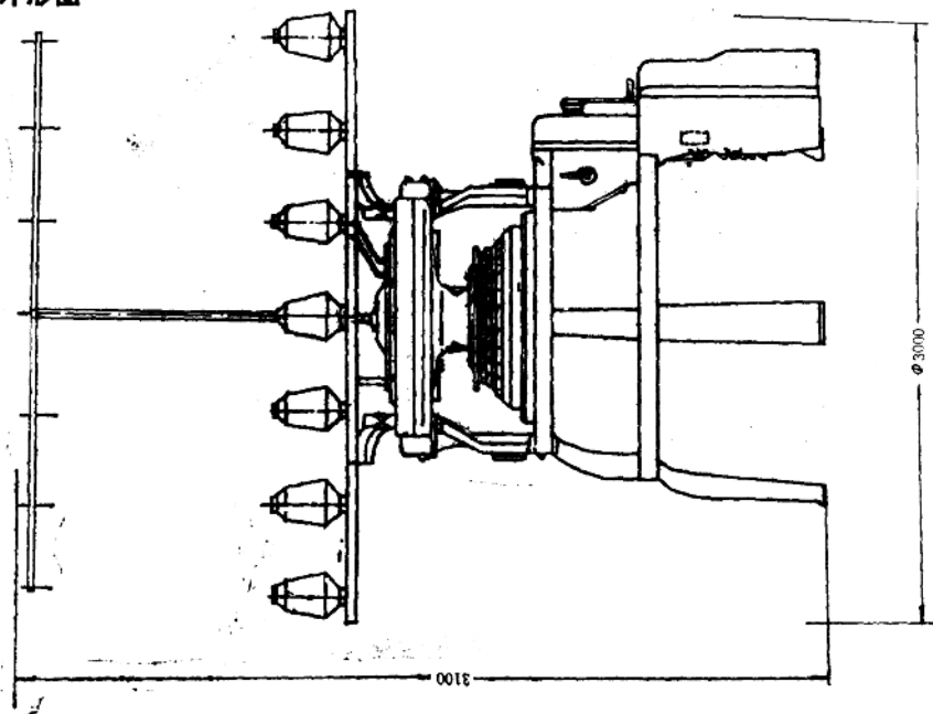
GE015型罗纹机外形图
