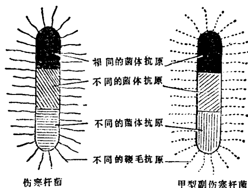
图3 伤寒杆菌和副伤寒杆菌菌体抗原和鞭毛抗原示意图
