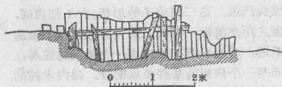
图三 木构遗迹二1号房剖面图
