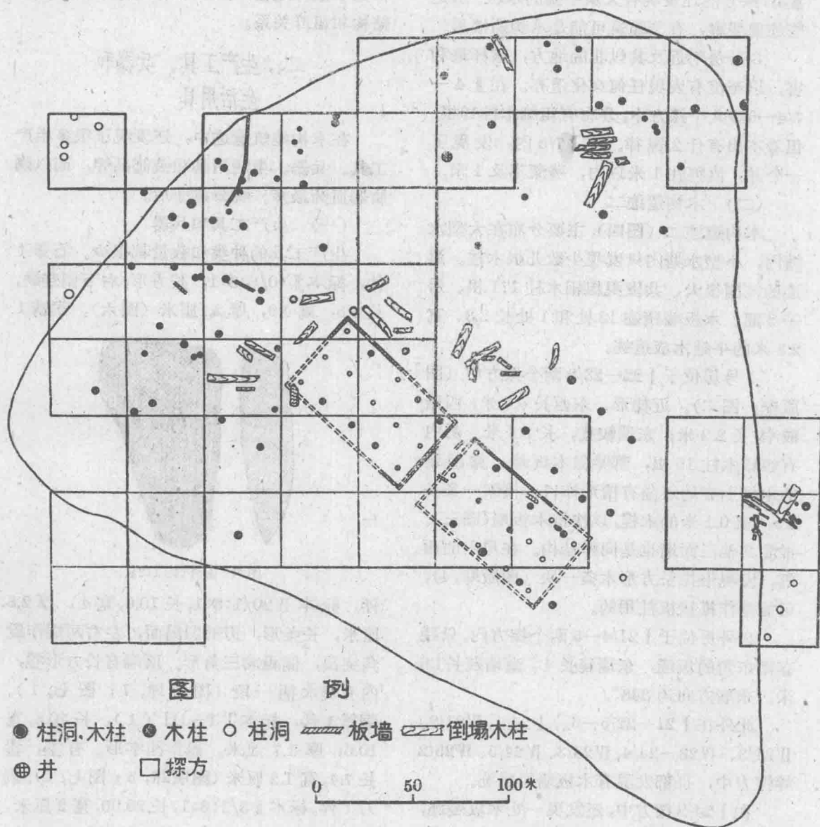
图五 木构遗迹一平面图(中型水塘内, 图内复原房子, 下为1号、上为2号)
