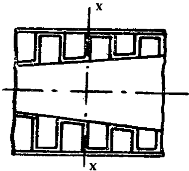
图 2-1 热力叶轮机机械叶片组的剖面 (原理图)
