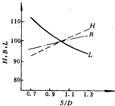
图 1-1 S/D 对外形尺寸的影响
