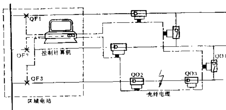
图 1-3 “不断电自动配电系统” 的部分接线
