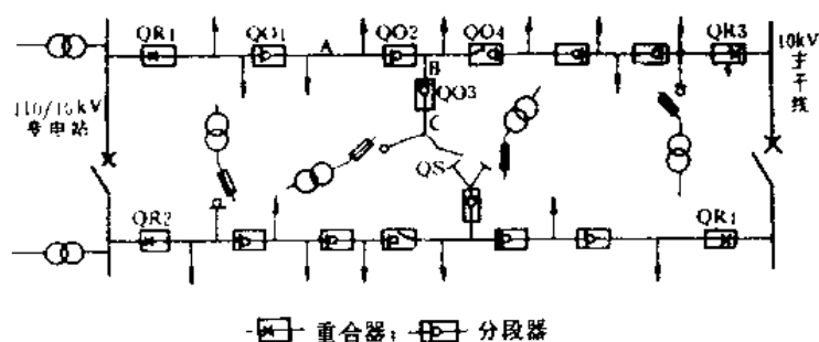
图 1-2 部分架空配电网结构示意图
