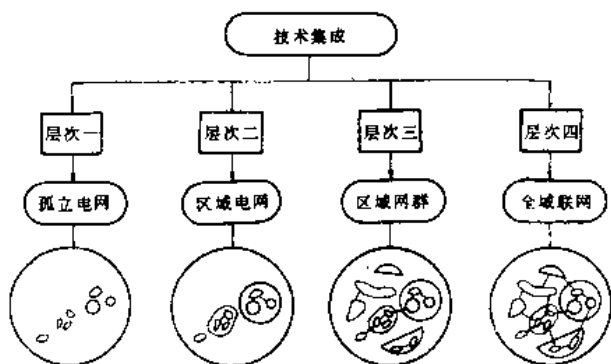
图 1 1 配电自动化的“层次”示意
