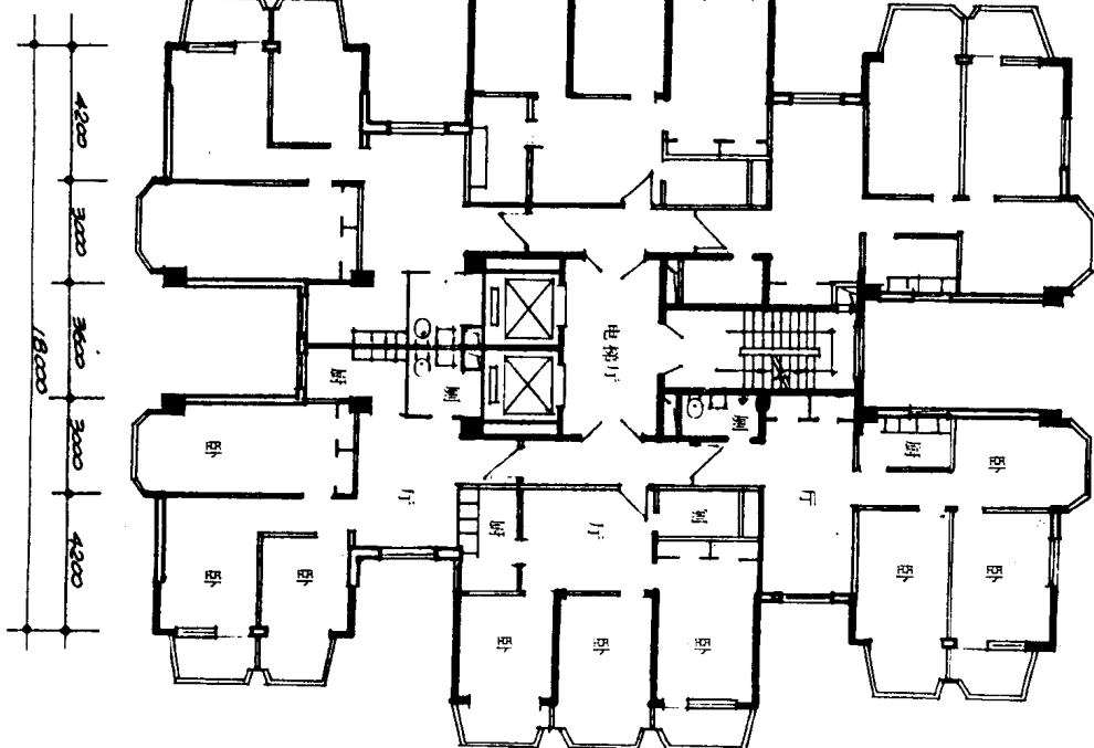
标准层平面
