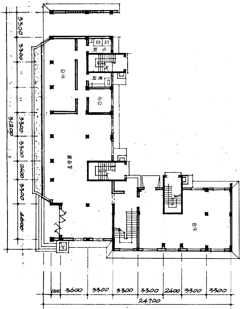
底层平面
