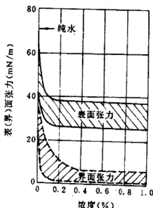
图 1-2 活性剂的表面张力和界面张力随浓度的变化范围(25°C)
