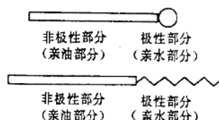
图 1-1 活性剂的分子结构
