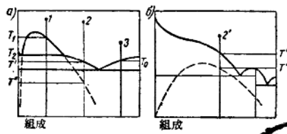
图 1 两种具有介穩分液作用的状态图 (虛綫表示介穩分層范围)
