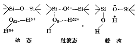
图6 水分子对网络硅原子的亲核侵蚀
