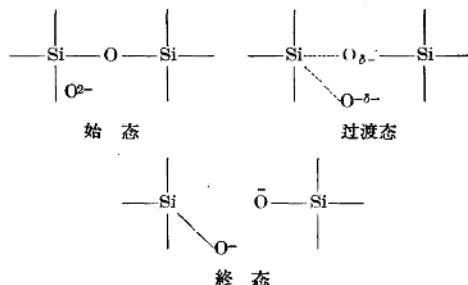
图3 氧离子对网络硅原子的亲核侵蚀
