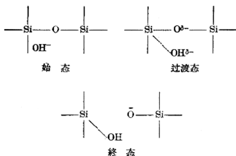
图4 氢氧离子对网络硅原子的亲核侵蚀
