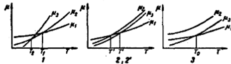
图2 相应于组成1, 2, 2', 3(见图1)时离子化学位 \mu 与温度的关系示意图
