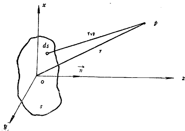
图1.2 计算孔径天线外场的坐标
