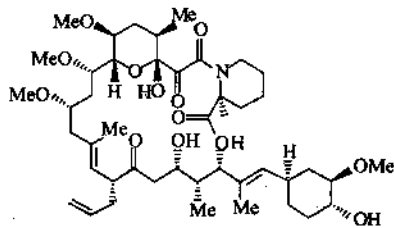
图 1-4 FK-506
