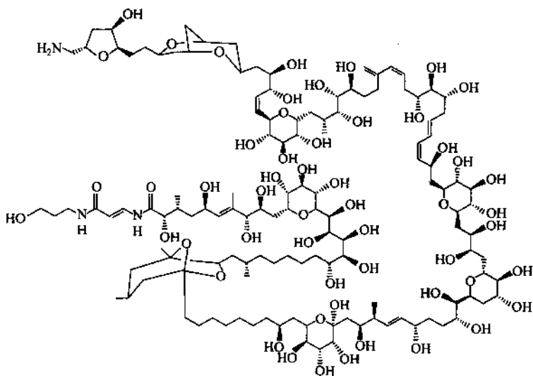
图 1-3 海葵毒素
