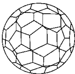
图 1-6 富勒烯
