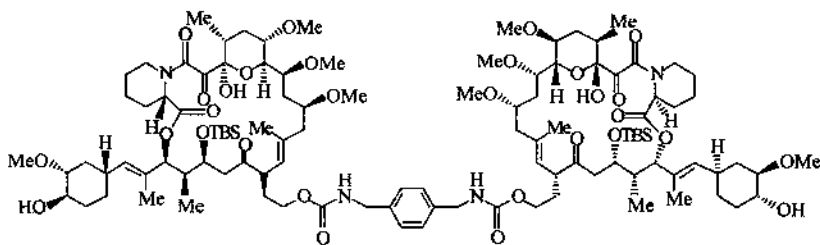
图 1-5 FK-1012
