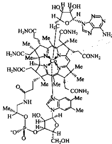
图 1-2 维生素 B 12
