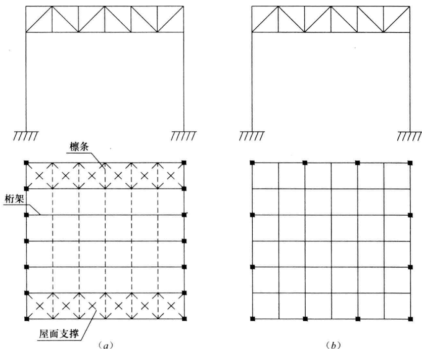
图 1.1.1 平面屋盖结构的不同做法
