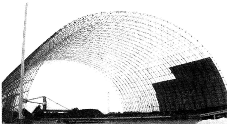
图 1.1.6 扬州电厂储煤库
