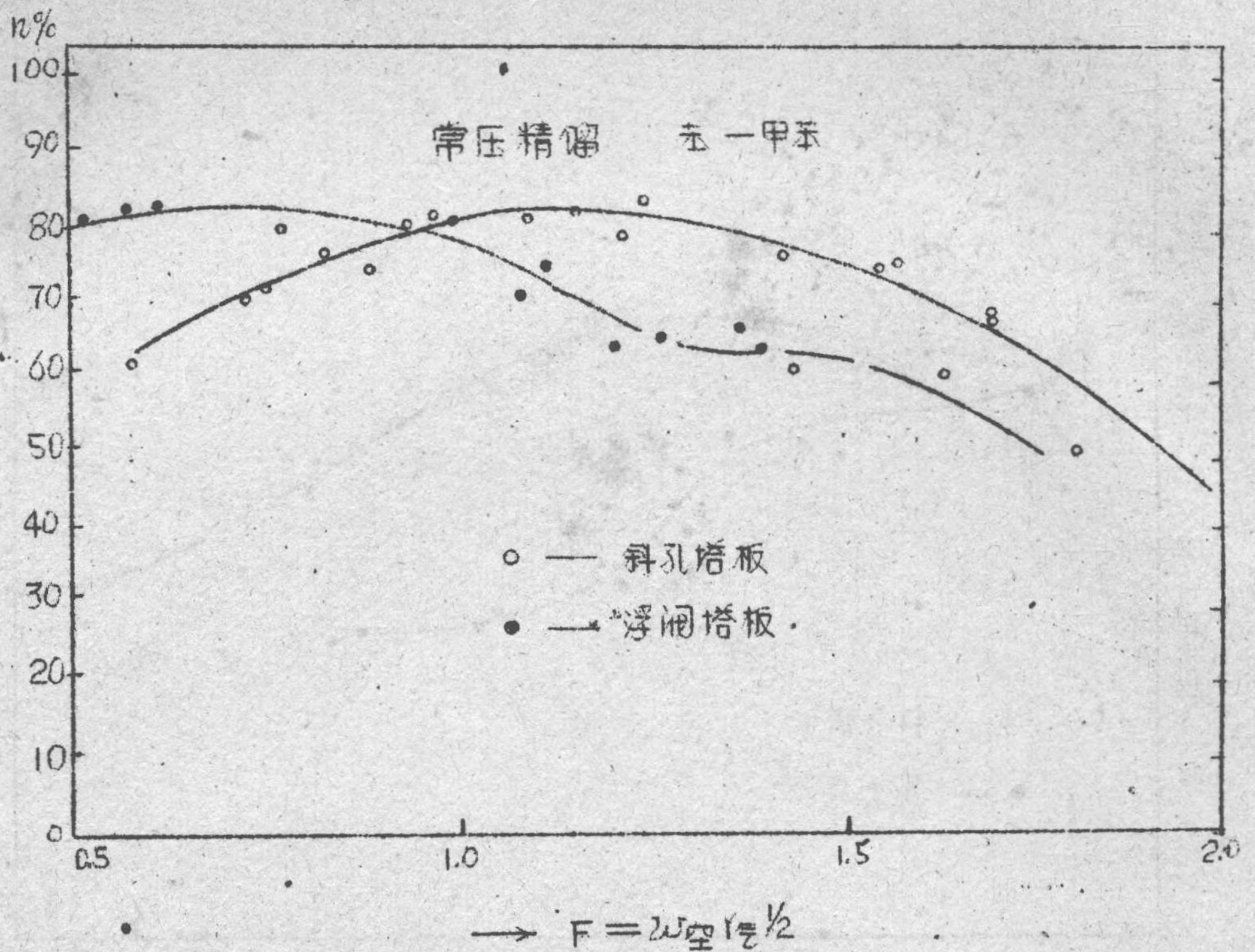
图 2-5 常压精馏塔板效率与动能因子 F 的关系
