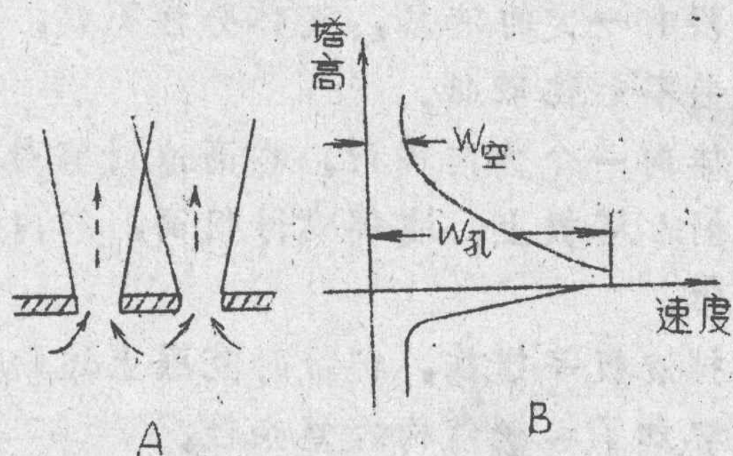
图 2-1 筛板上体流通截面与速度分布
