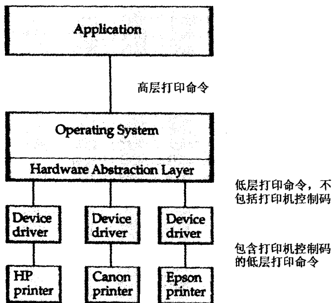
图 1-3 设备驱动程序增加了特定设备代码
