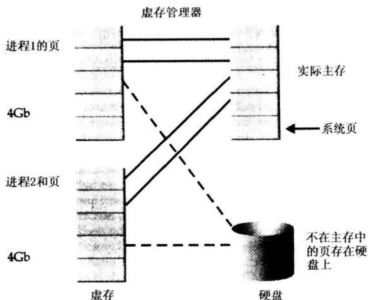
图 1-2 虚存管理
