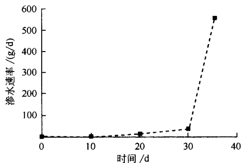
图 2-1 淀粉微生物法膜材的渗水速率与时间曲线
