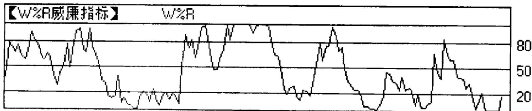
图1-1 威廉指标示意图
