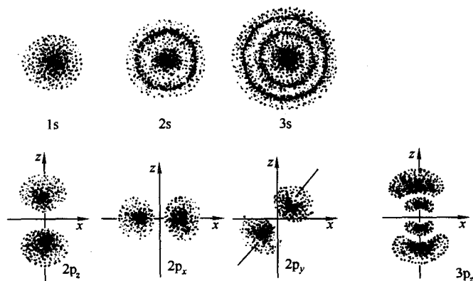
图 1-4 电子云示意图
