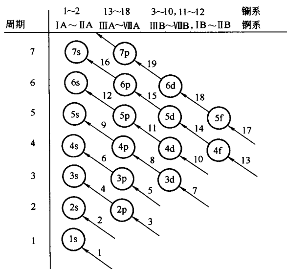
图 1-8 电子填充顺序图
