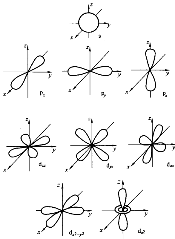
图 1-5 电子云角度分布图
