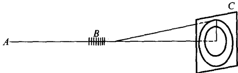
图 1-1 电子的衍射现象
