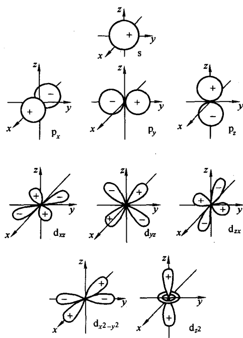
图 1-3 s, p, d 轨道角度分布图
