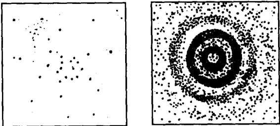
图 1-2 电子衍射实验结果示意图
