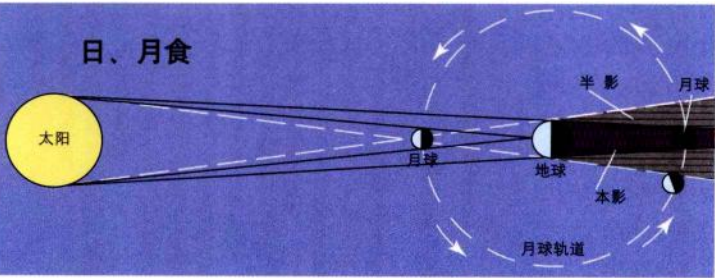
▲ 日食与日、月、地的关系
