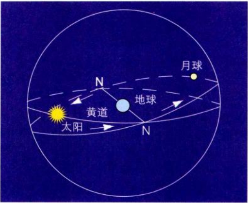
▲ 月球轨道界面
