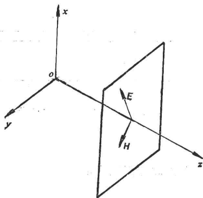
图1-4 沿 z 方向传播的平面电磁波
