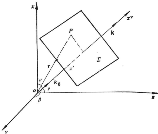
图1-5 一般坐标系下的平面波
