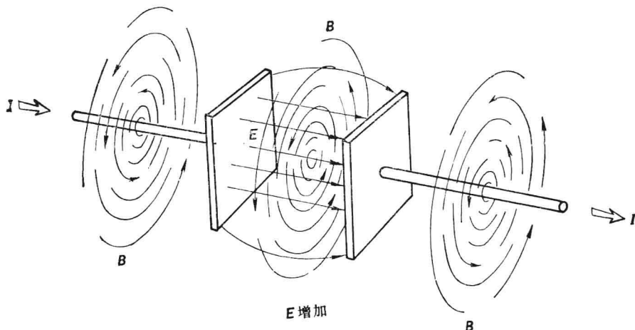
图1-2 电容器充电和放电时两极板间变化电场产生磁场
