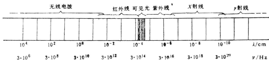
图 1-3 电磁波谱
