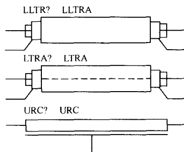
图 1.10 传输线元件
