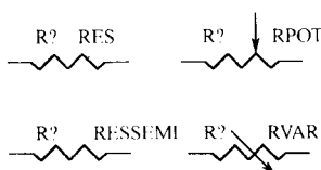
图 1.1 电阻元件
