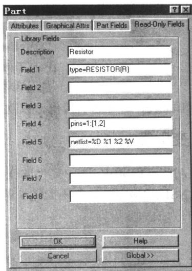
图 1.3 只读框
