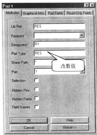
图 1.2 属性框
