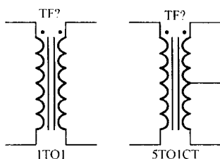
图 1.7 变压器元件
