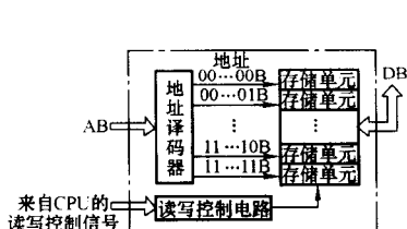
(a) 存储器结构示意图
