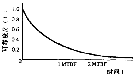
图1.2 可靠度曲线
