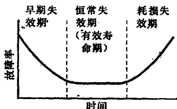
图1.1 故障率随时间变化曲线
