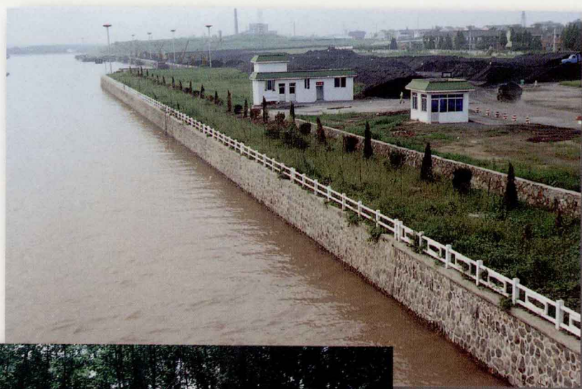
直立式护岸
