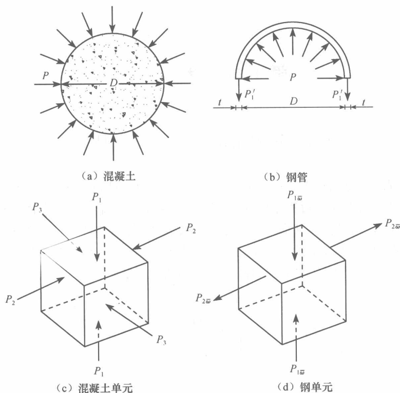
图 1.2 钢管和混凝土的受力状态图
