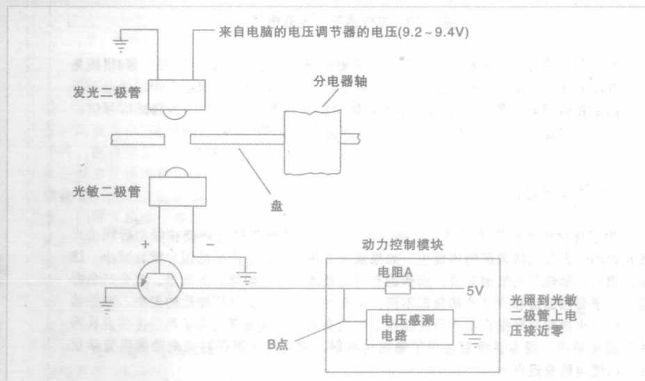
图2-19 分电器中的光电传感器
