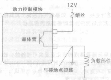
图2-1 计算机为执行器供电，与接地点短路可能会损坏计算机的驱动器
