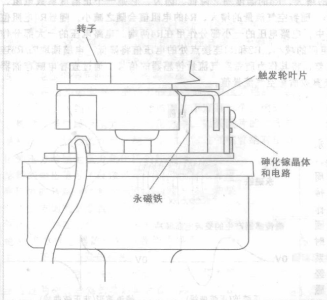
图2-15 霍尔效应开关
