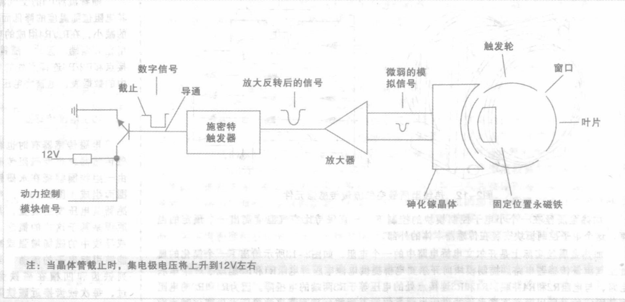
图2-16 霍尔效应开关电路
