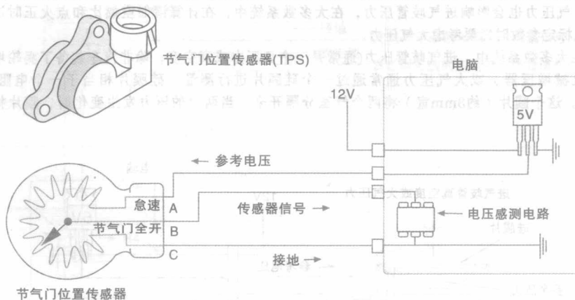
图2-8 用作节气门位置传感器的电位器
