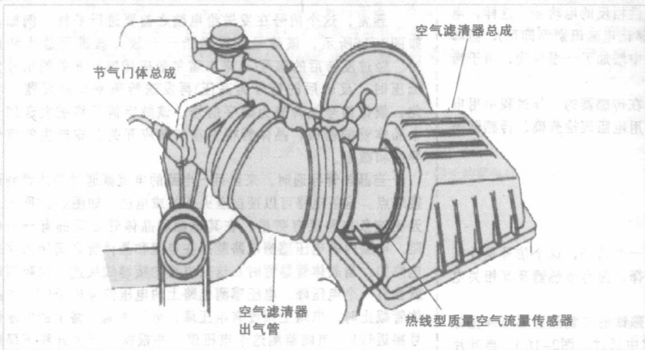
图2-11 热线型质量空气流量传感器的位置
