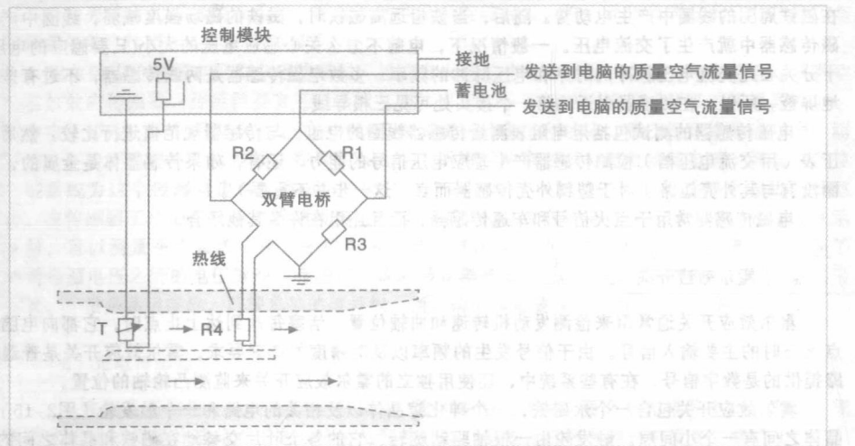
图2-13 质量空气流量传感器电路
