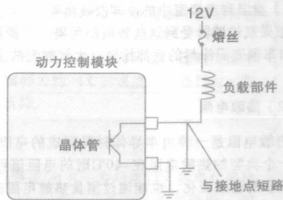
图2-2 计算机完成执行器的接地电路，与接地点短路执行器通电，但不会使计算机过载
