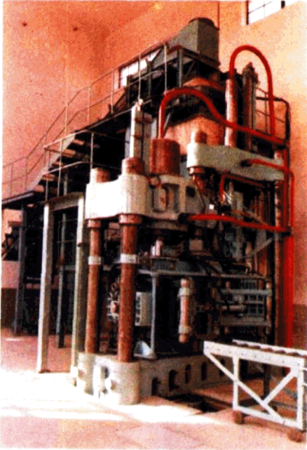
▲500吨饲草打包机
