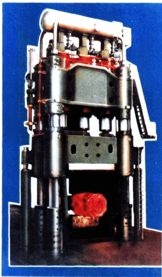
▲6000吨锻造水压机
