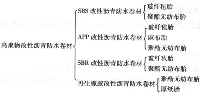
图 1-4 高聚物改性沥青防水卷材主要类型及品种
