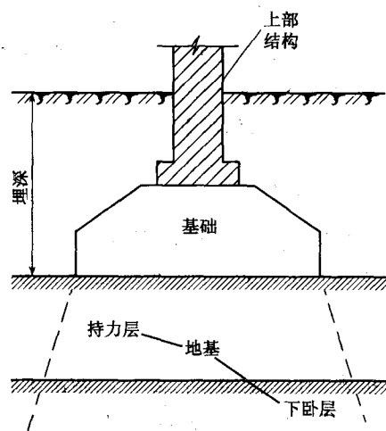
图 1-1 地基基础示意图
