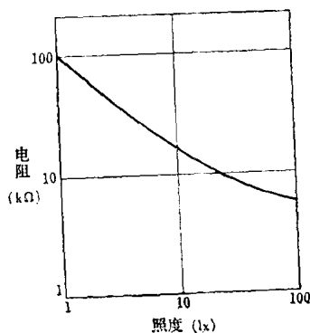
图 1.5 CdS的特性
