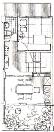
平面参考图
