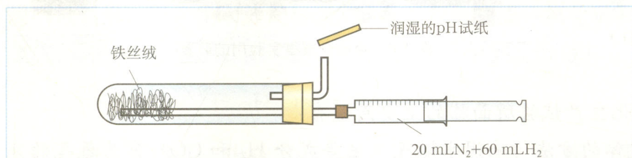
图 1-5 合成氨的实验装置
