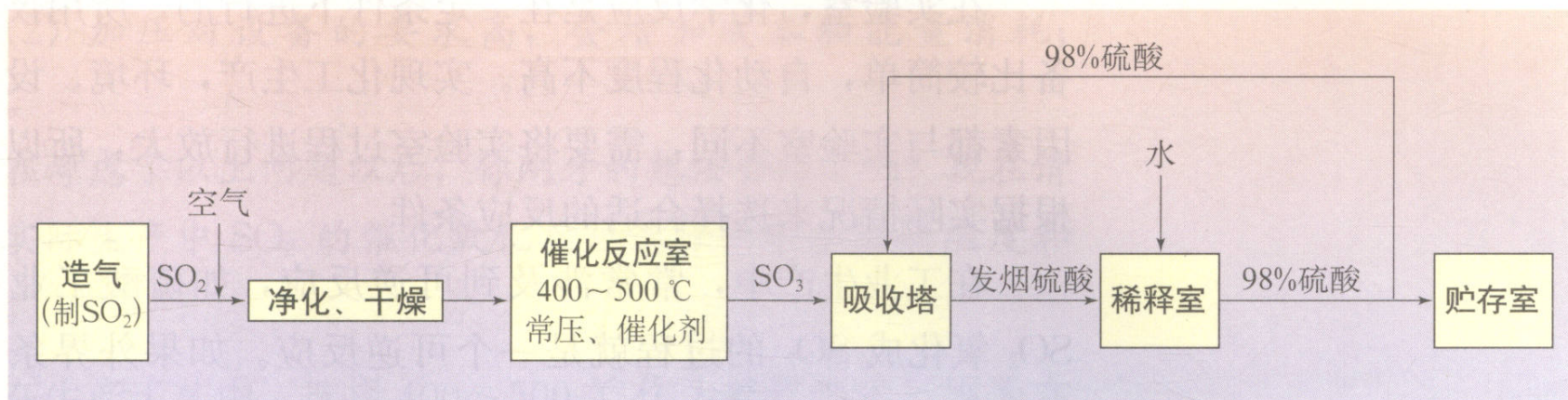
图 1-2 硫酸工业流程
