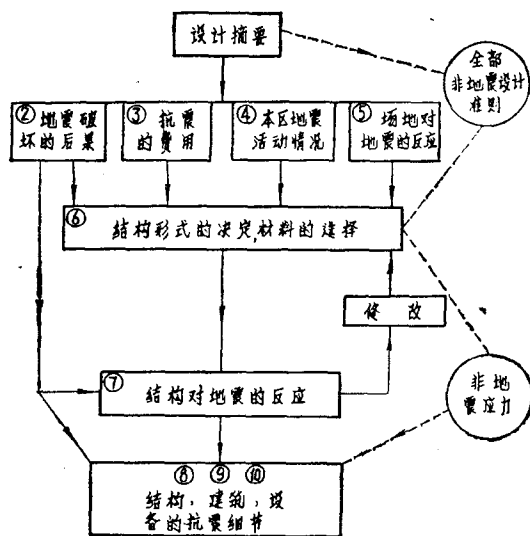
建筑物抗震设计的简单流程
