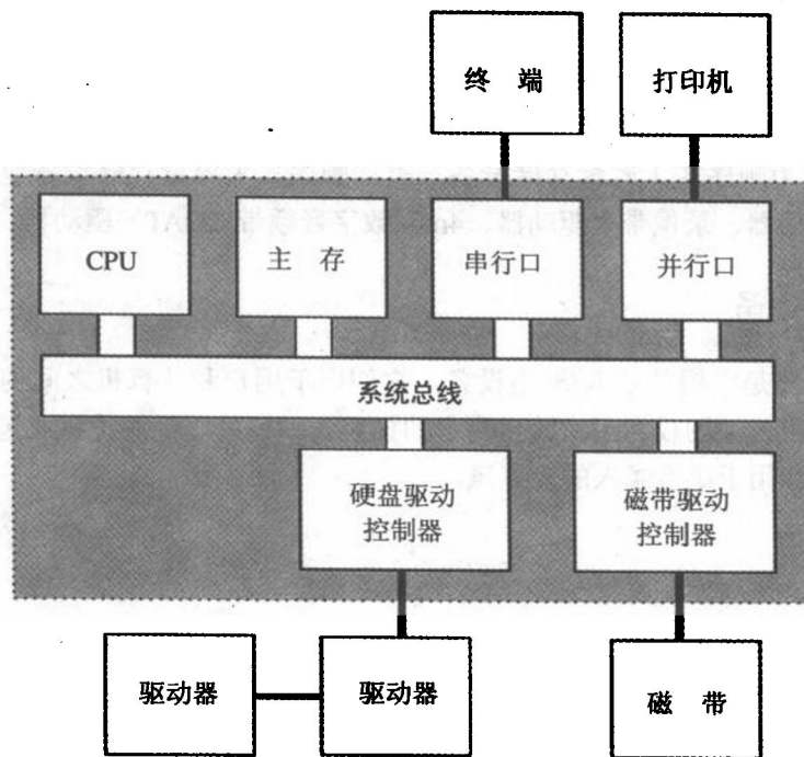
图 1.1 带有外围设备的计算机系统
