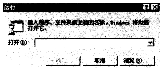
图 1-2-1 “运行”对话框
