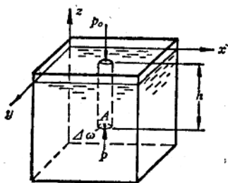
图 1-3 静止液体中压强分布
