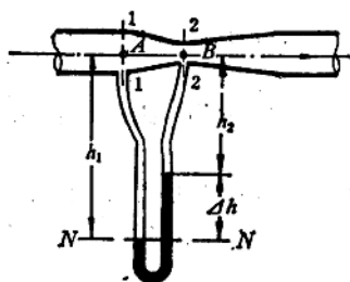
图 1-7 文丘里流量计
