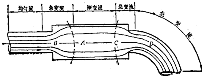
图 1-11 均匀流和非均匀流
