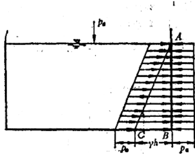
图 1-4 水池壁相对压强分布图
