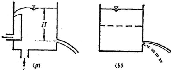
图 1-9 恒定与非恒定流动
