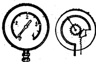
图 1-8 弹簧压力表
