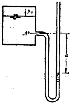
图 1-5 测压管
