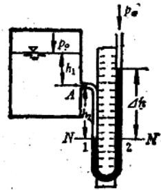
图 1-6 水银测压计
