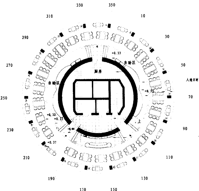
塔楼一层旋转餐厅平面图
