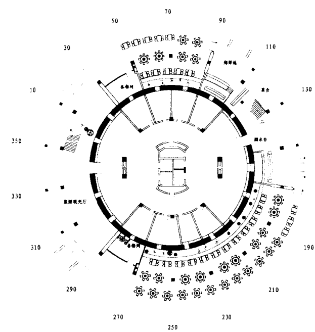
塔座一层平面图
