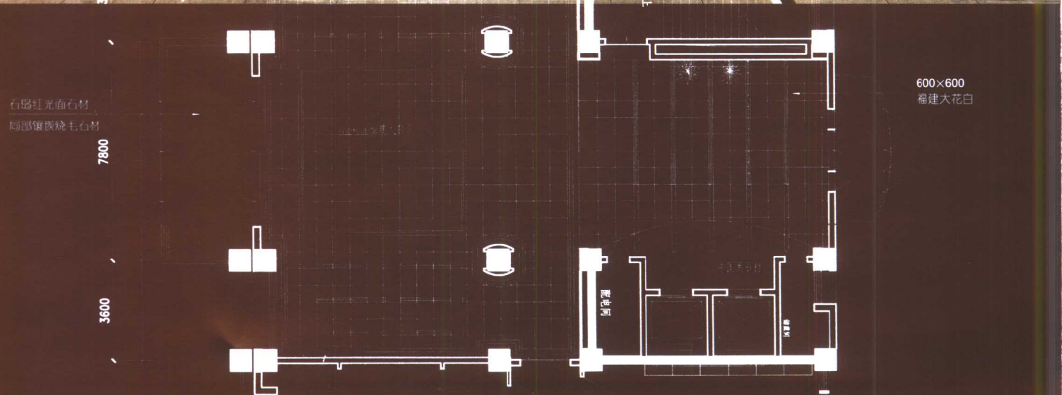
一层大堂及电梯间平面图
