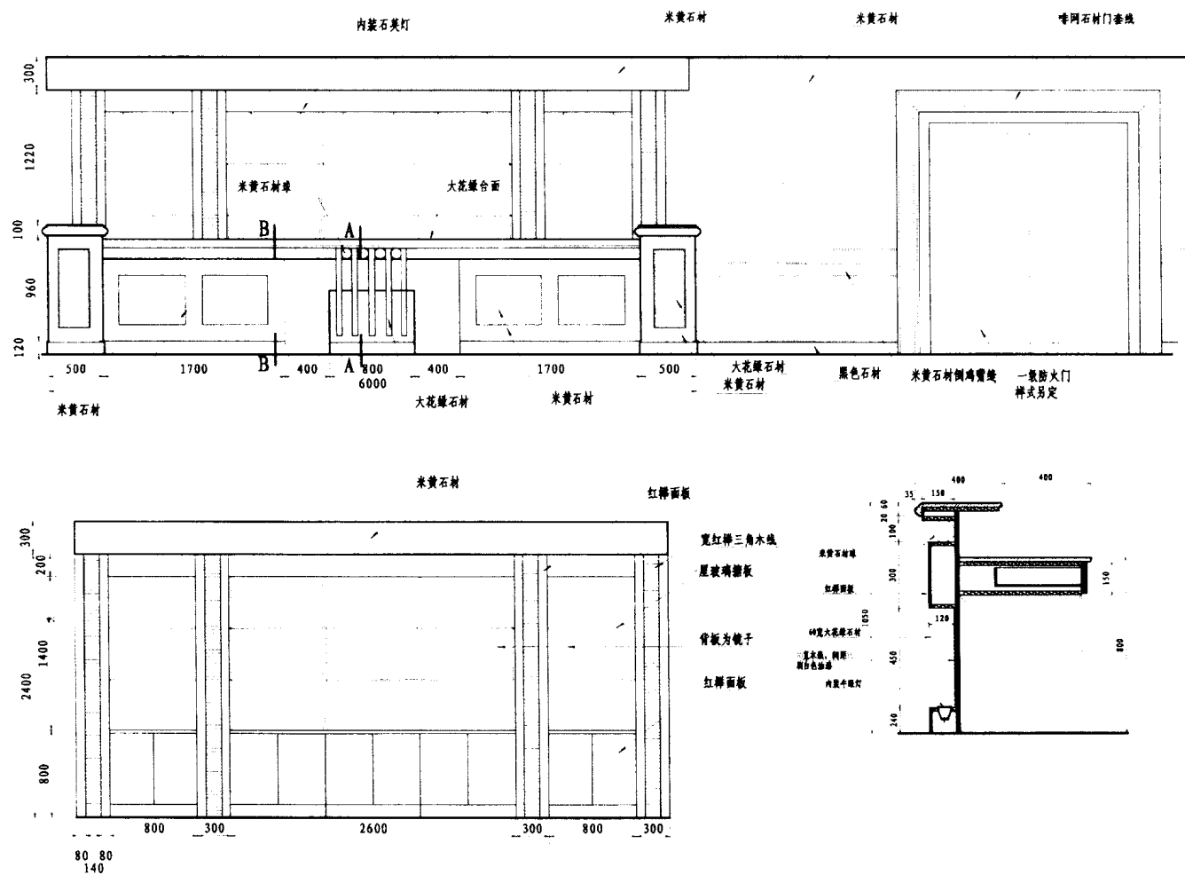
一层服务台立面及剖面图
