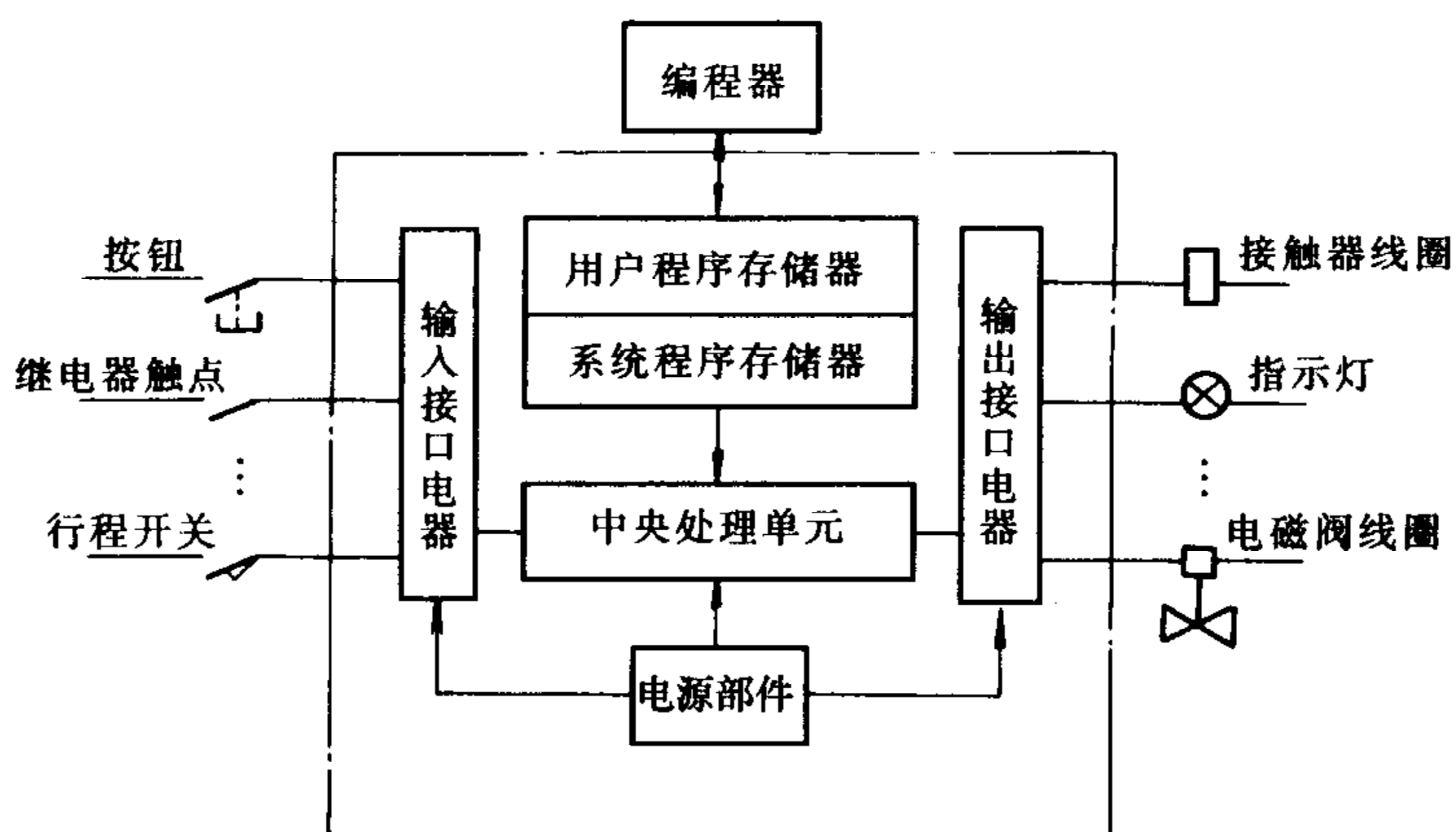
图 1-1 PLC 的组成
