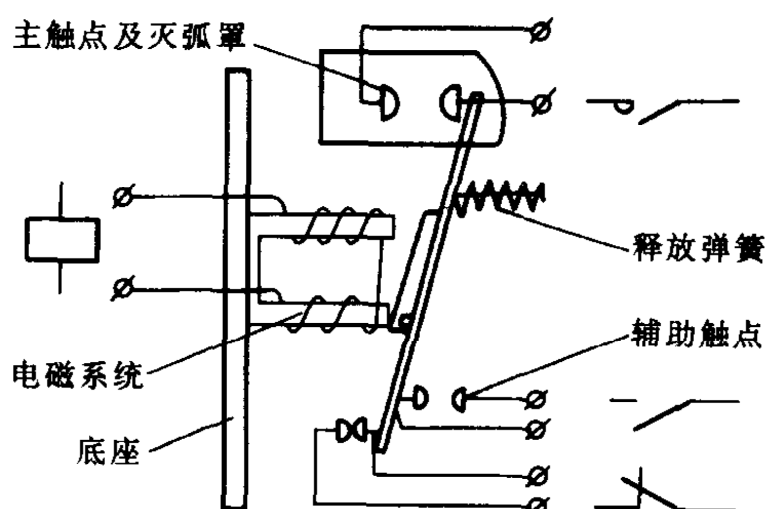
图 1-2 接触器工作原理
