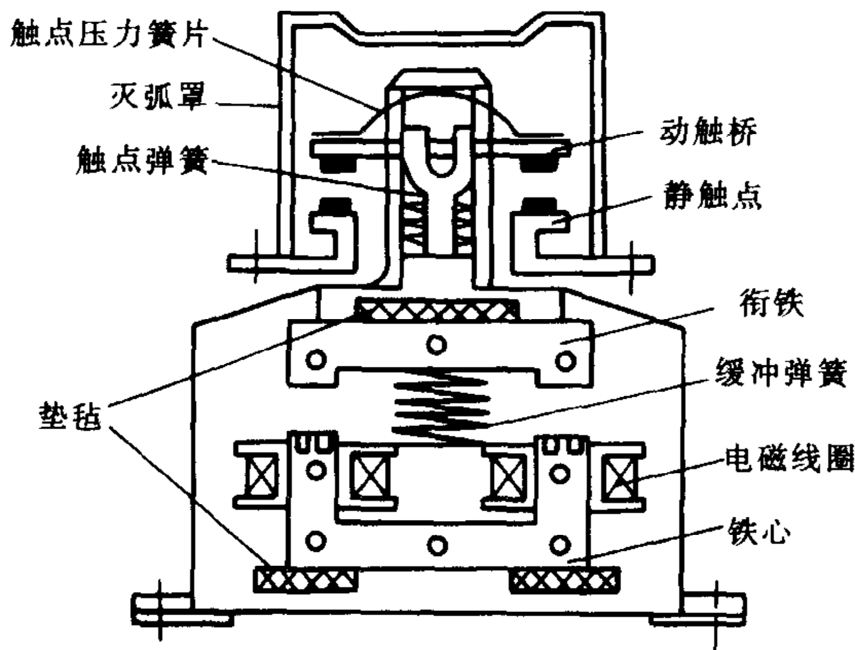
图 1-4 CJ20-63 型交流接触器的结构示意图
