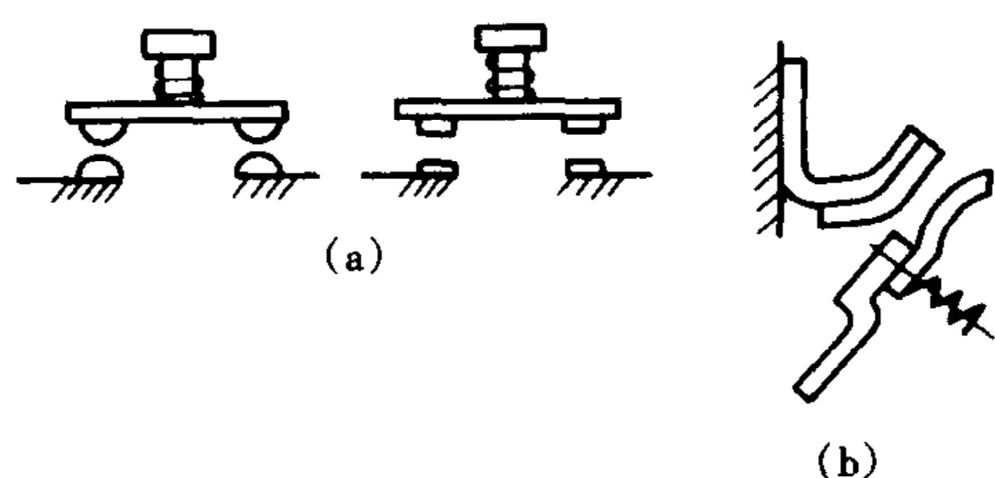
图 1-3 触点结构型式 (a) 桥式触点; (b) 指型触点
