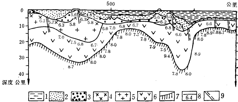
图4 横过萨哈林岛(库页岛)一千岛的地壳剖面(据 Тугезов, И. К. 1975)
