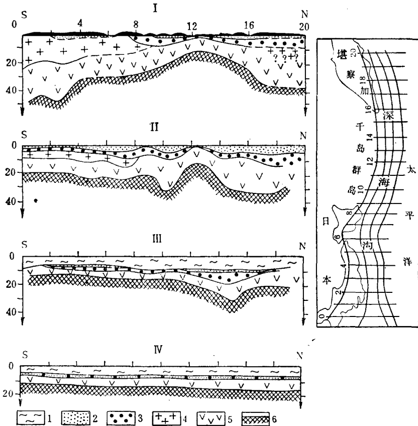
图5 从日本—千岛—堪察加岛弧向太平洋地壳结构变化图(据 Тугезов, И. К. 1975)
