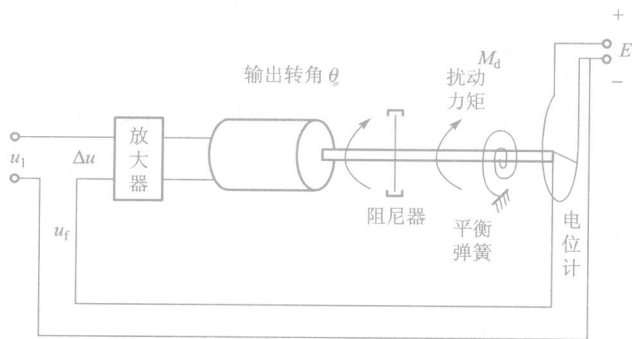
图 1-3 闭环控制系统
