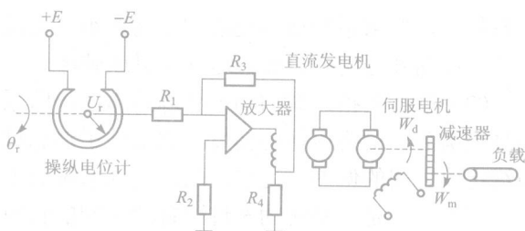
发电机-电动机调速系统
