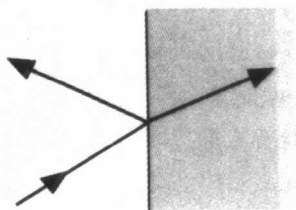
左右的折射率不同的情形
