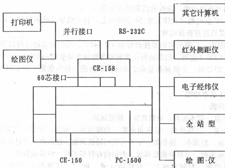
图 2-1 PC-1501 与外围设备的连接图
