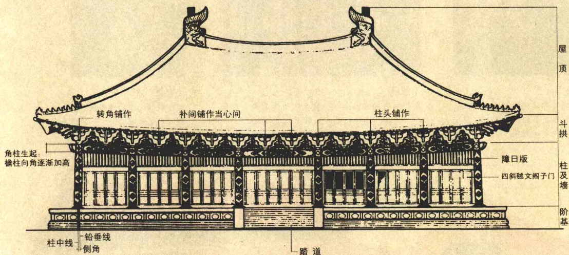
↑北京故宫太和殿立面处理示意图
