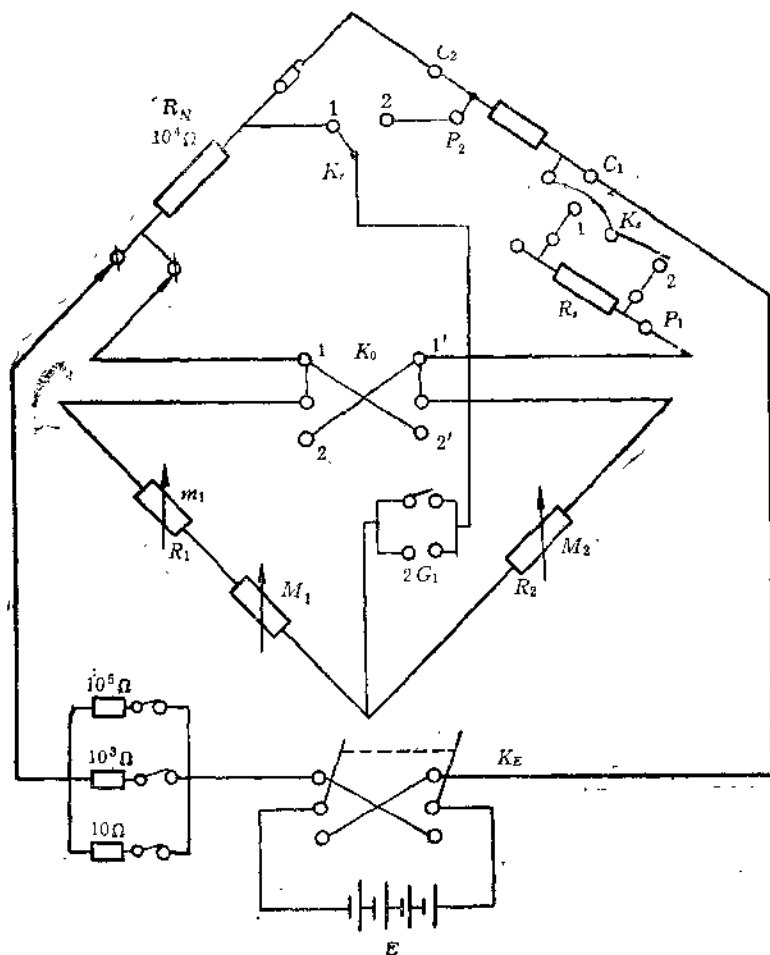
图2 比较电桥比例臂检定原理线路图
