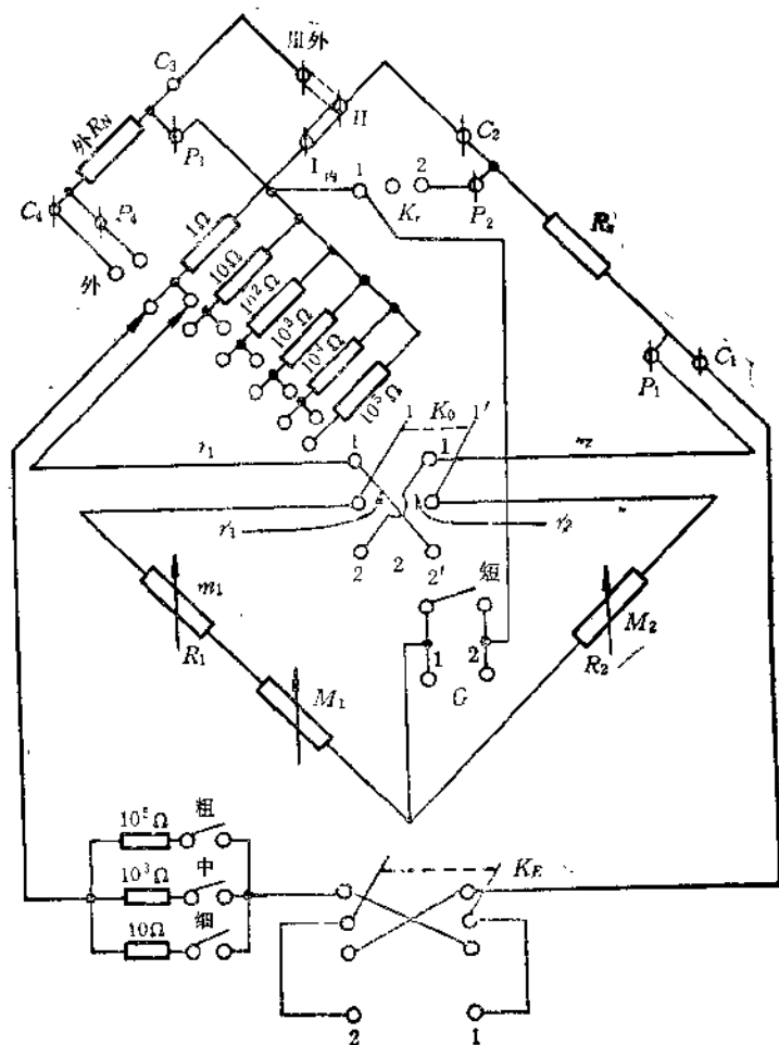
图1 比较电桥原理线路图
