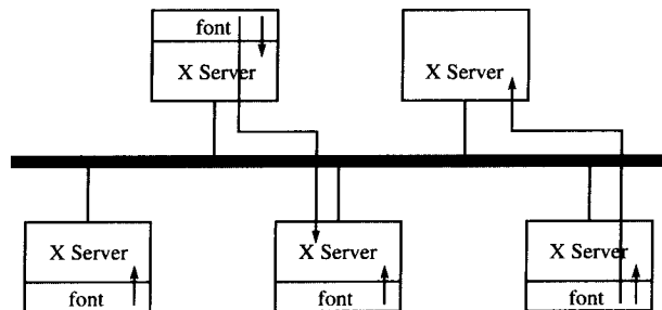
图 1-2 X font server
