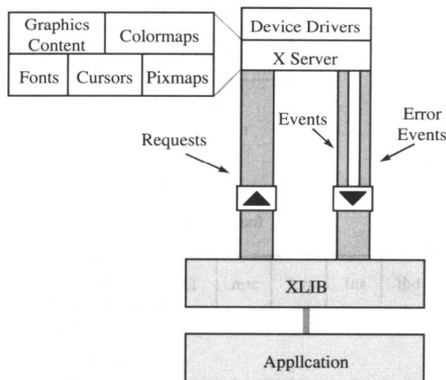
图 1-4 X Server 与 X Client 间的交互
