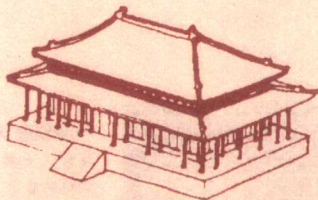
重檐庑殿顶
