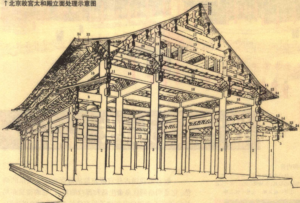
↑故宫太和殿梁架结构示意图
