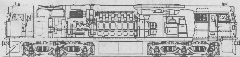
圖 1.4 工程圖
