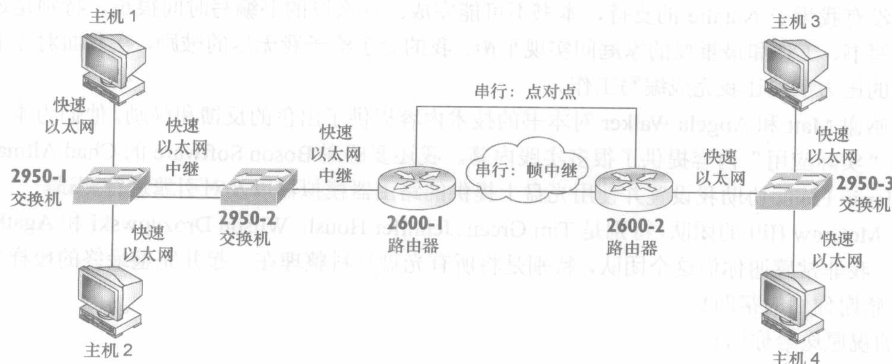
图 1 实践练习的基本网络拓扑
