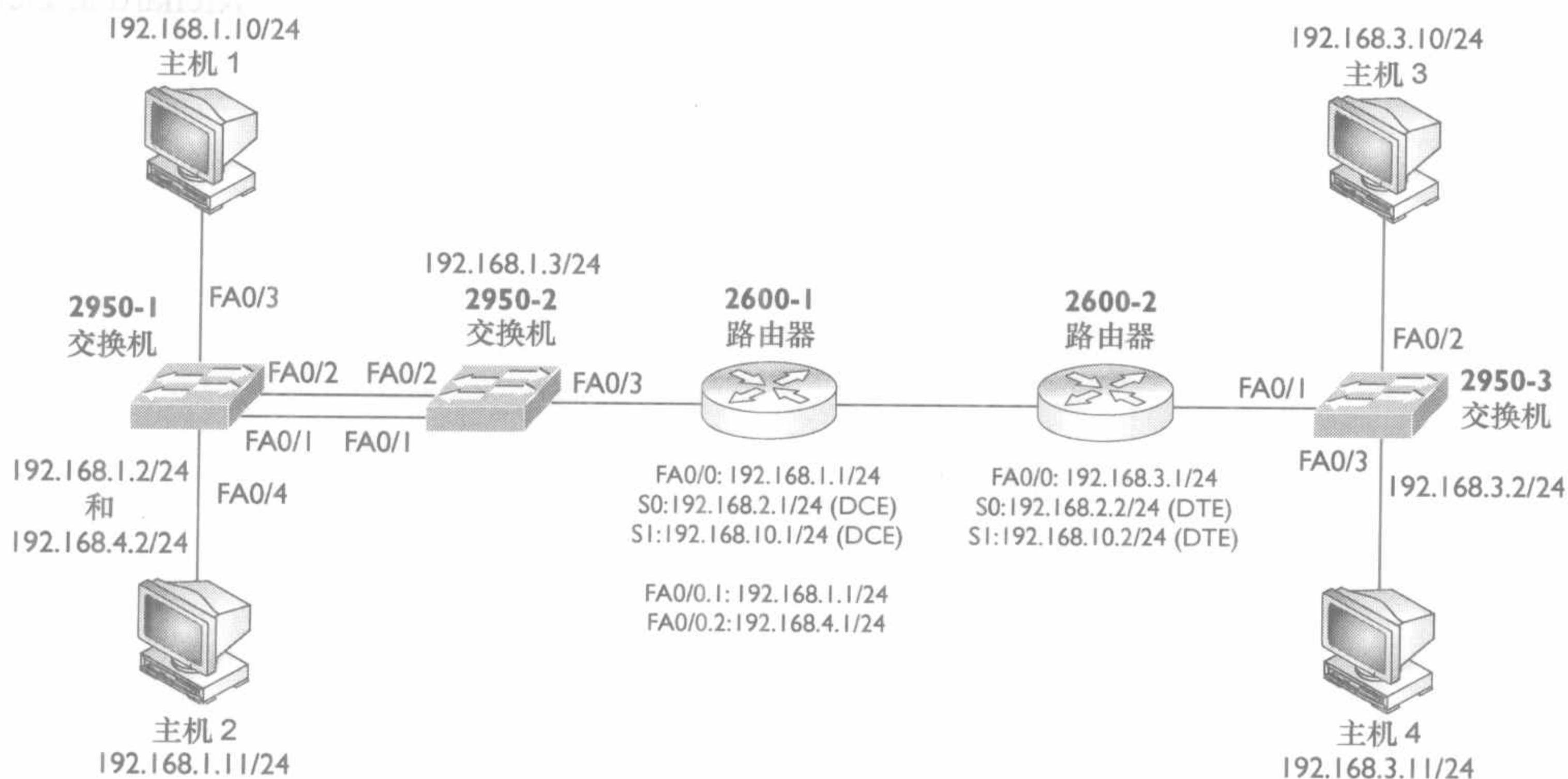
图 2 实践练习的基本网络拓扑寻址
